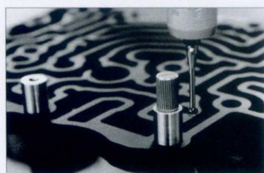
使用三次元測定螺絲孔位置
