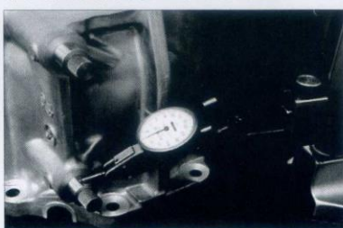
使用高度計測定螺絲孔位置
