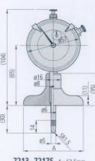
7213, 7217S An ø3.5mm 7214, 7218S An ø1.5mm
